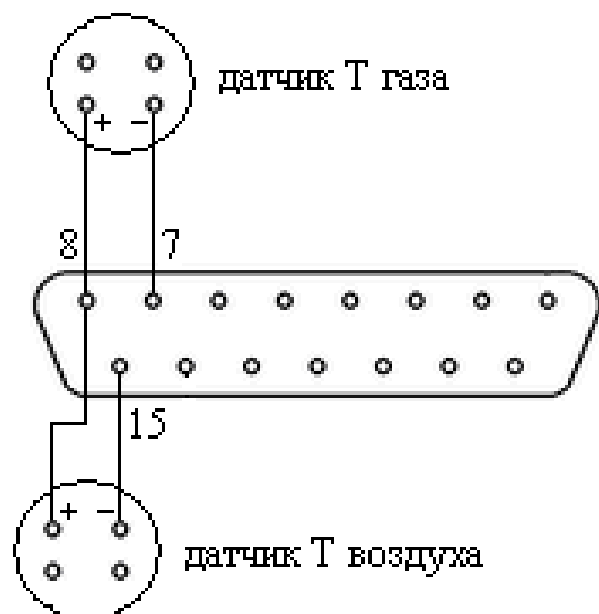
Подключение датчиков температуры Рис. 2
